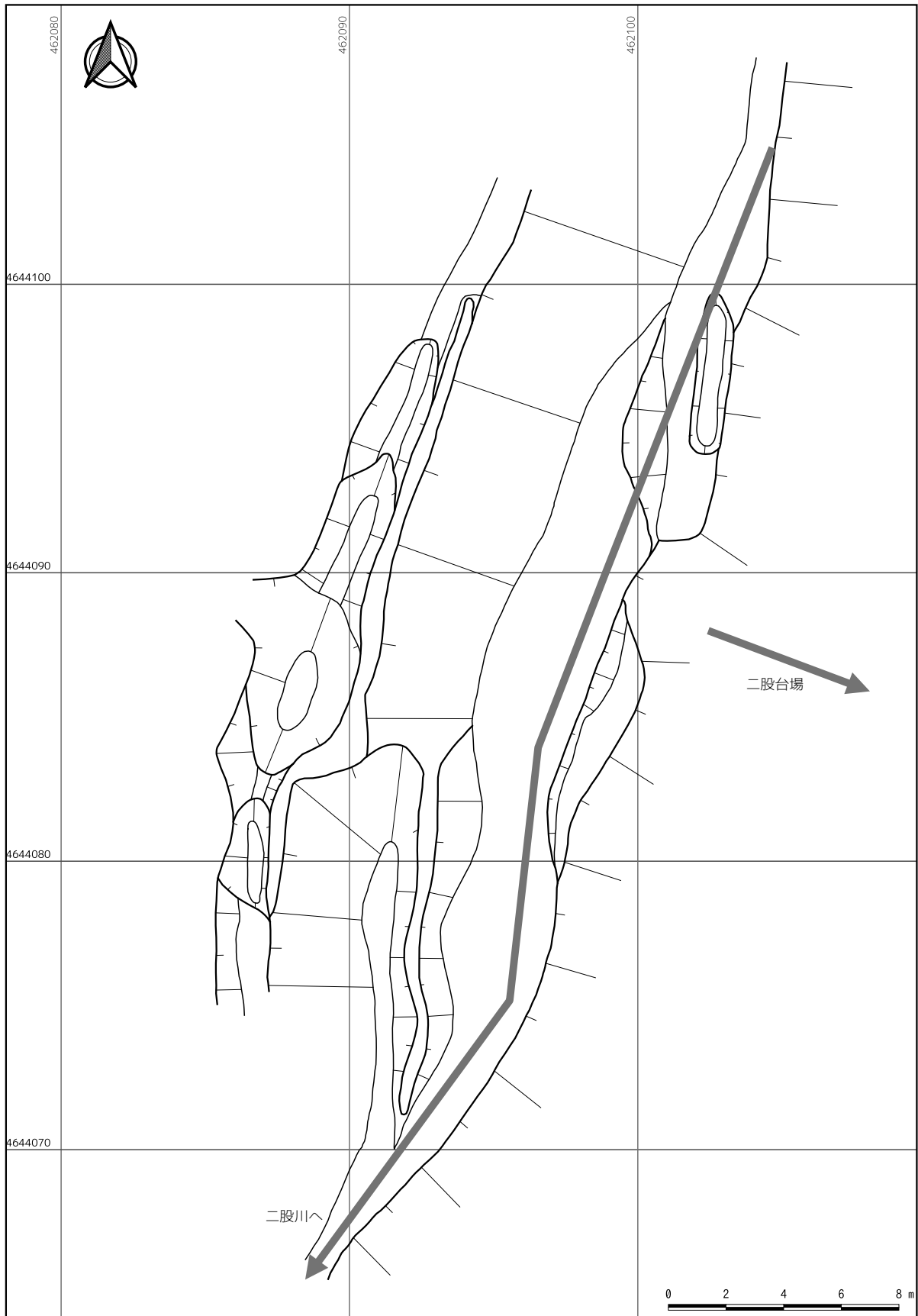
図5 S01 平面図
