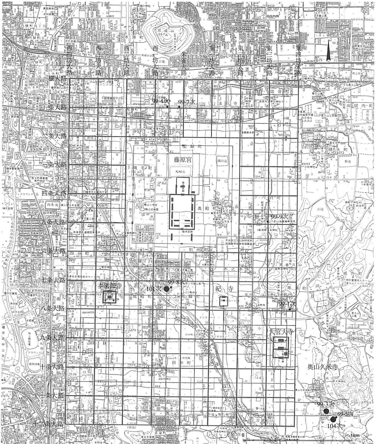
図15 藤原京の調査位置図 1:20000
