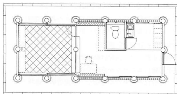
朱雀門案内所平面図 (1:150)
