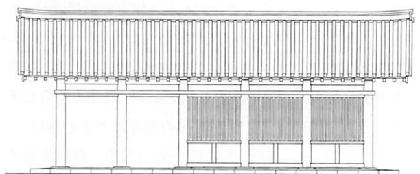
同左南立面図 (1:150)
