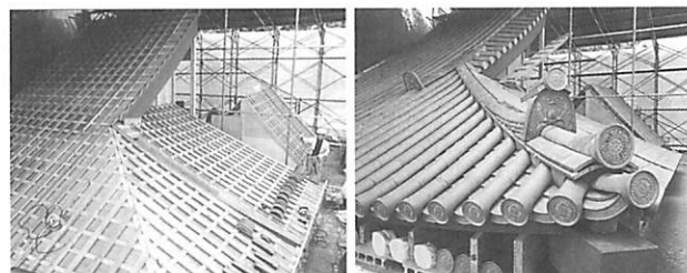
屋根廻り試し葺き用実大模型の製作
