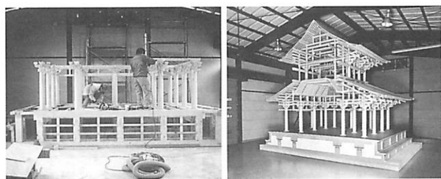
五分の一構造模型の製作
