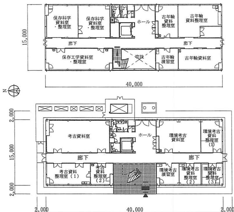
文化財資料棟 一階平面図（600m 2 下） 二階平面図（566.91m 2 上）
