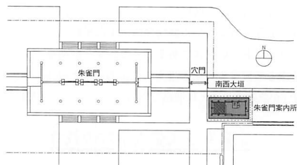
朱雀門案内所配置図 (1:1000)
