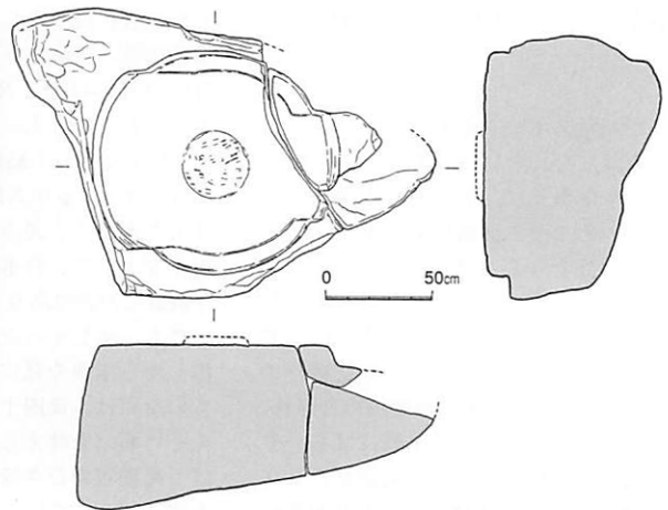
図78 寄贈礎石実測図 1:40
