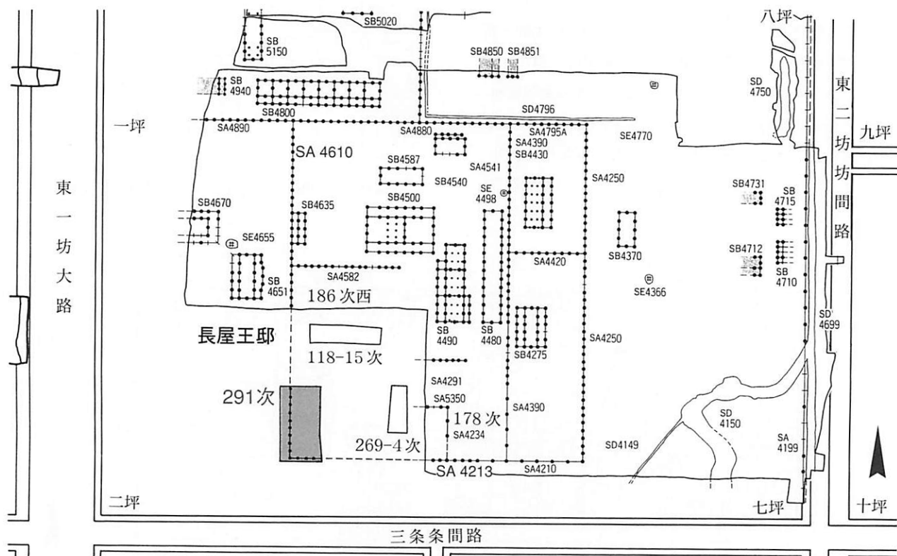
図77 第291次調査 発掘位置および周辺遺構（A期）配置図
