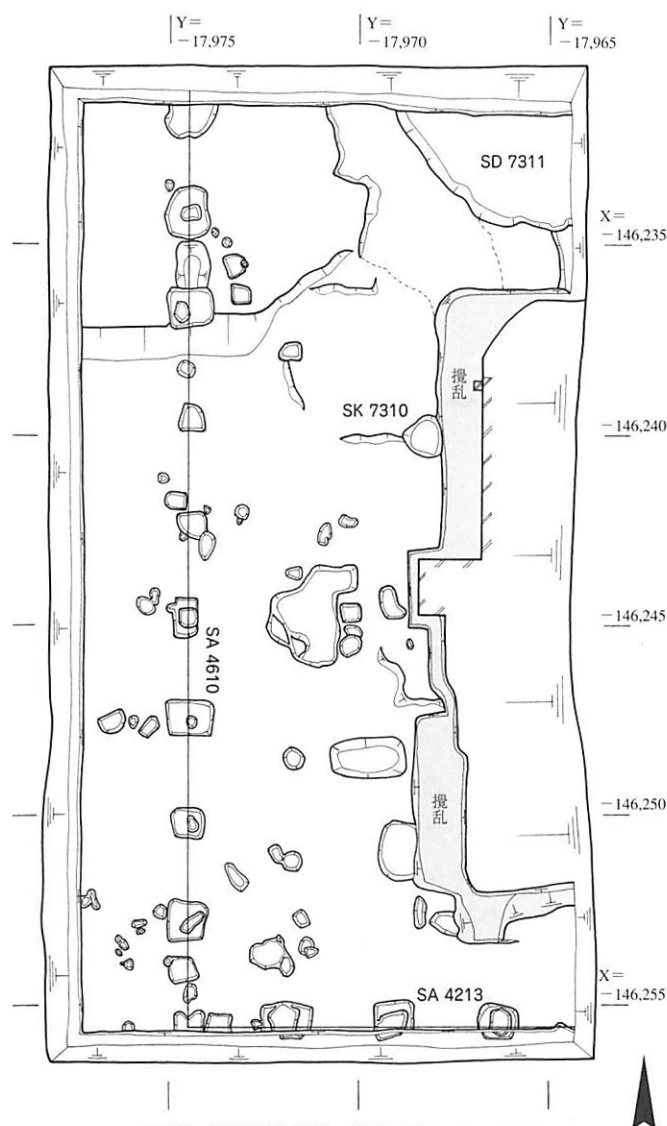
図78 第291次調査 遺構平面図 1:200
