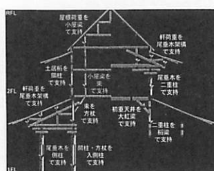
初重 二重 架構の支持機構
