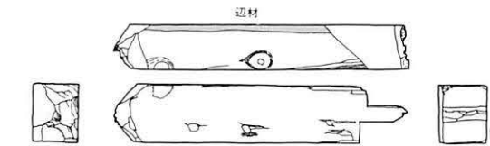
図2 SX277出土建築部材実測図 1：30
