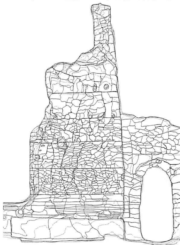
西北小寺院 仏塔周壁(部分) 1:70
