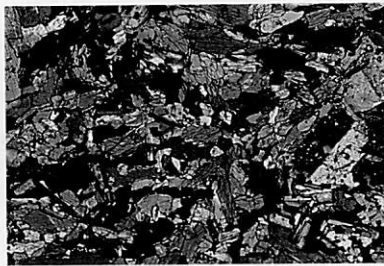
+ニコル [×30]
