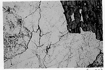
-ニコル [×30]
