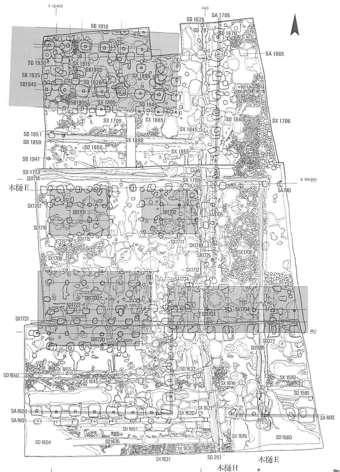
石神遺跡調査遺構図（第10・11・12次）およびA期主要遺構 1：300
