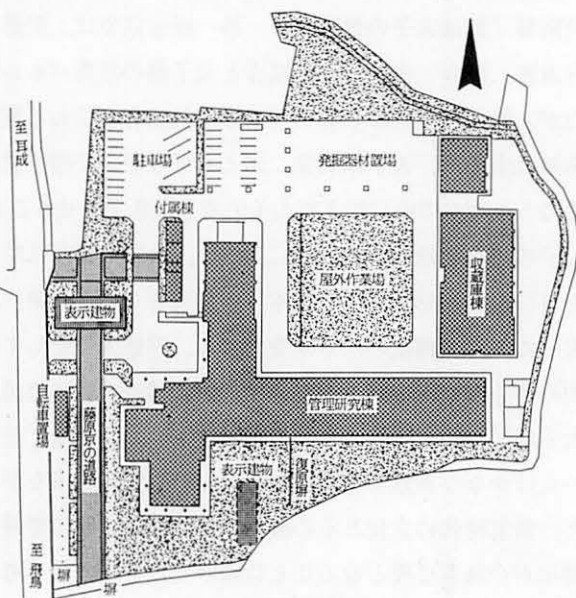
庁舎敷地平面図
