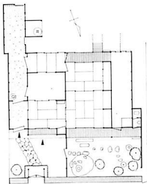
東家平面図（社家の1例）
