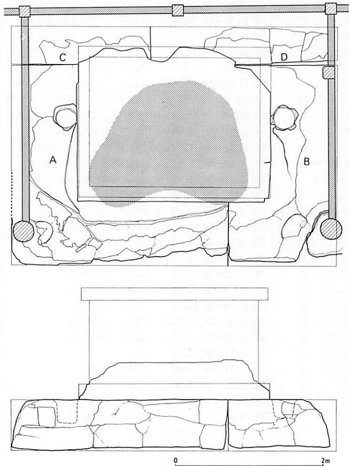
飛鳥寺旧本尊台座復原図
