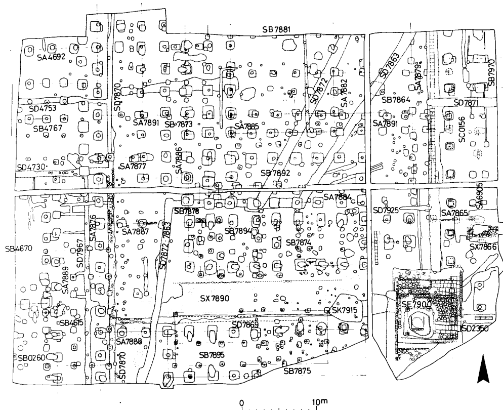
第1図 第78次南遺構配置図
