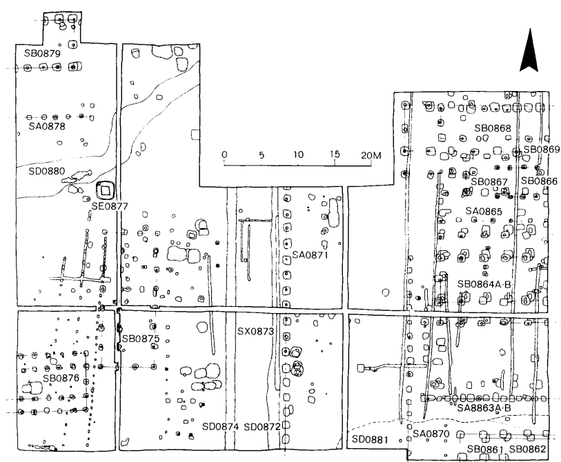
第12図 83次調査遺構配置図
