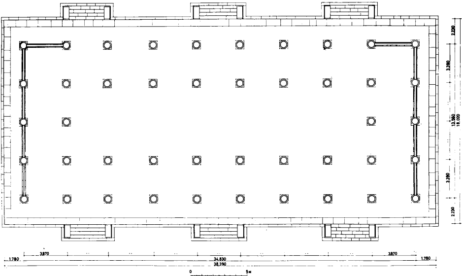
平面図
