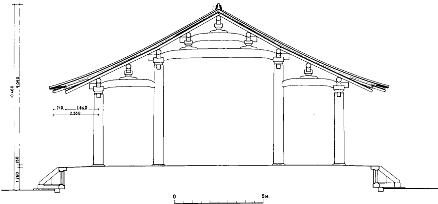
断面図
