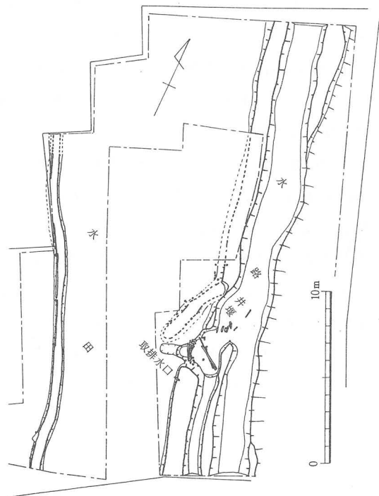
第3図 板付遺跡夜日式期の水田址 (原図『板付遺跡概報』)
