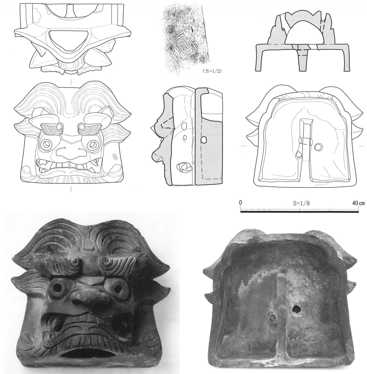
第7図 鬼面瓦4（多神社 拝殿）
