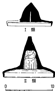
図4 分類の範例
