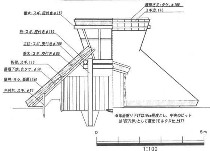
図1 弥生時代の復元住居 見取り図
