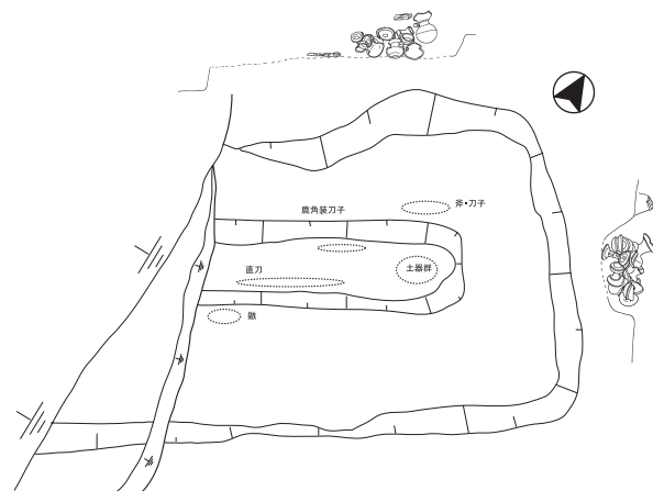
第10図 明気2号墳埋葬施設 出土状況略図（1：60）
