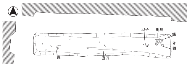
第4図 立岡山6号墳埋葬施設(1:60)(報告②に加筆)
