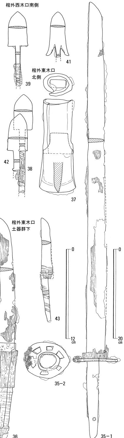
第 11 図 明気 2 号墳 出土遺物 (36 ~ 43 1 : 3 35 1 : 5)
