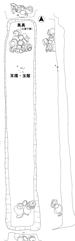
第13図 明気4号墳埋葬施設出土状況図(1:50) (報告②に一部加筆)
