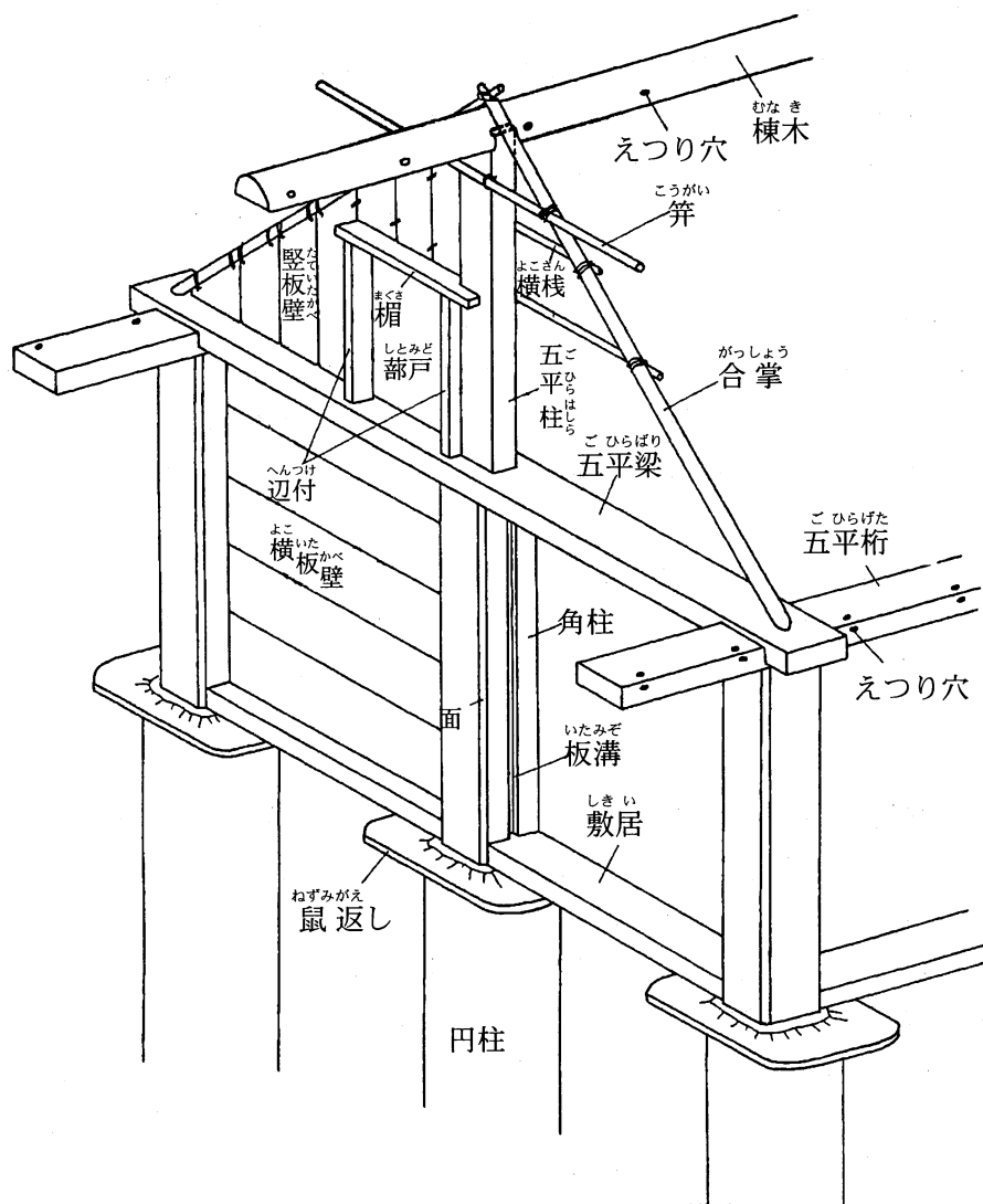
圖1 高床建築切妻側面構造模式圖
