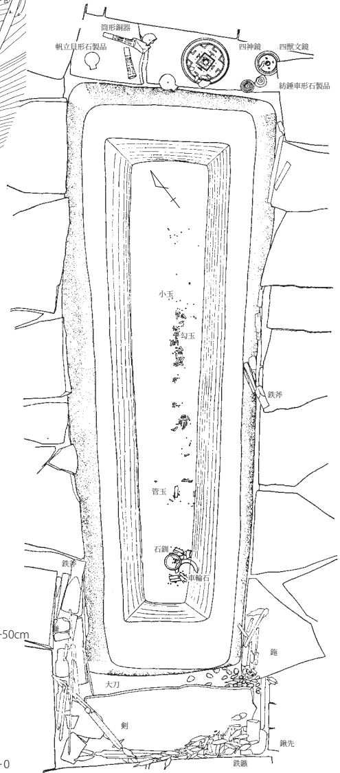
三池平古墳 遺物出土状況図
