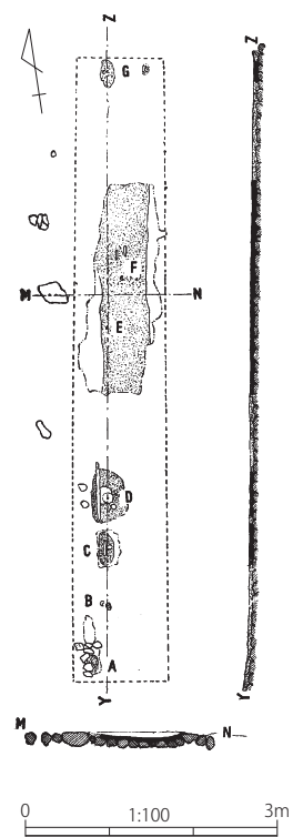
東坂古墳 埋葬施設実測図
