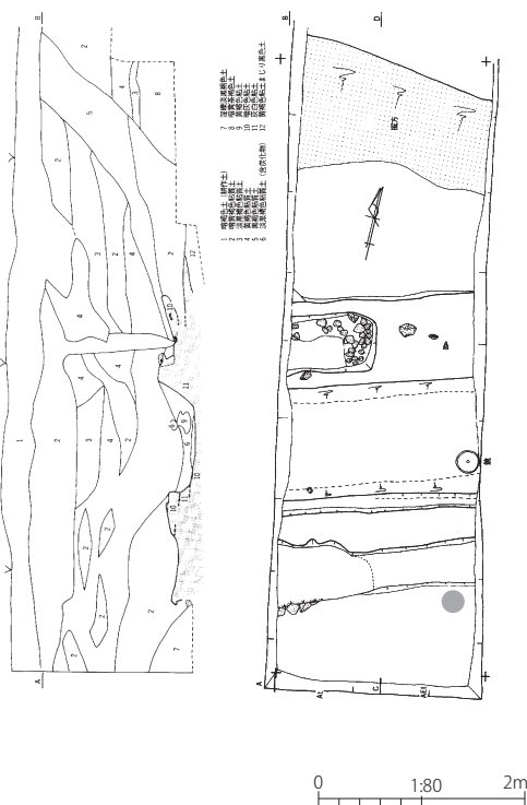
午王堂山3号墳 埋葬施設実測図
