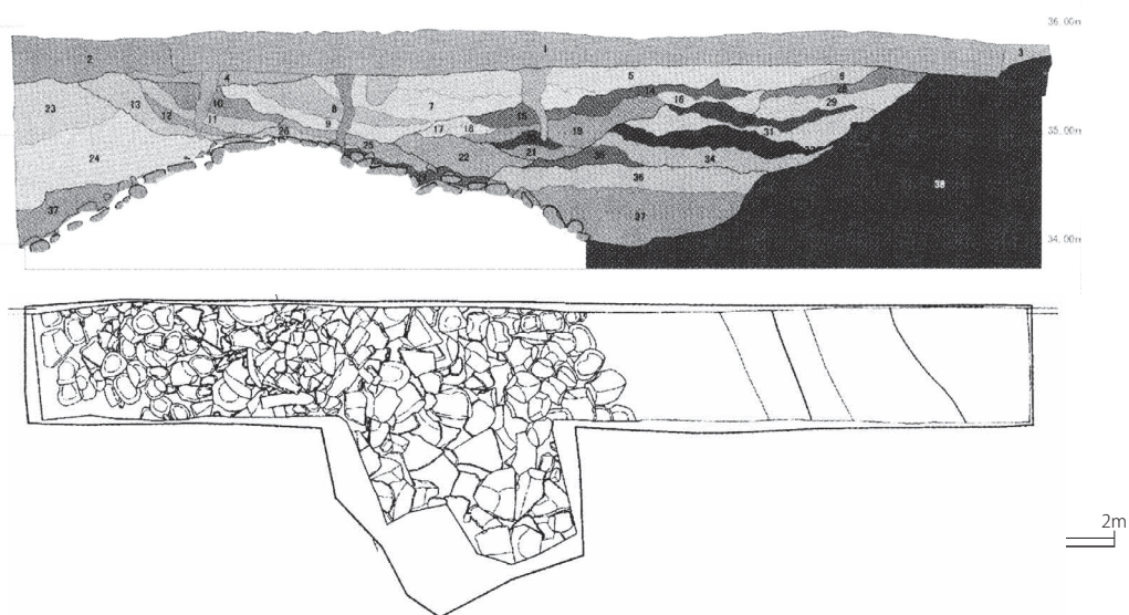
縦穴式石槨 平面図・断面図
