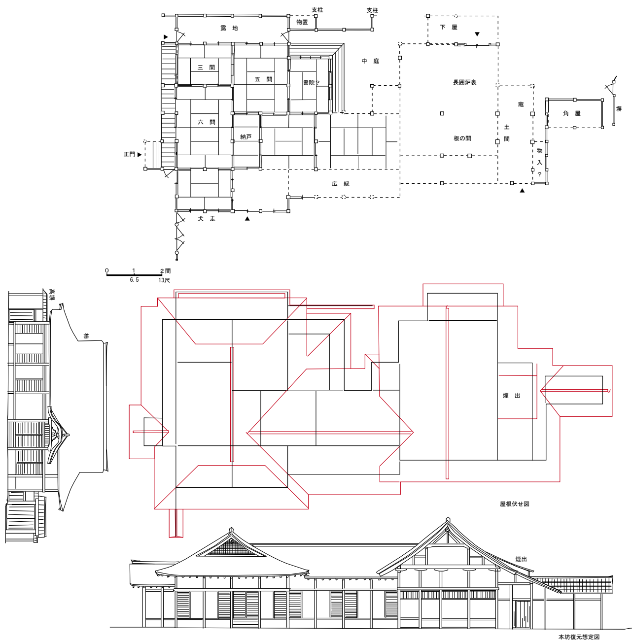
図 3-24 本坊SBO3復元平面・立面図（東・南面）
