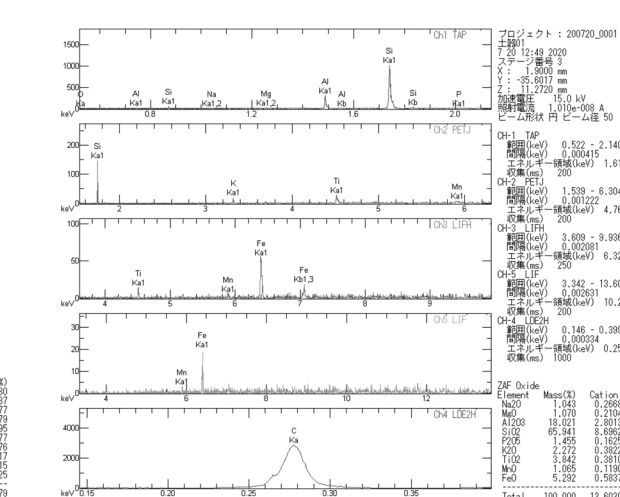
第146図 土器No. 1の定性分析 左：C含有 右：C除去
