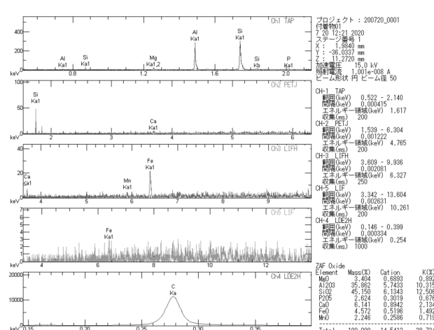
第144図 白色物質No. 1の定性分析 左：C含有 右：C除去
