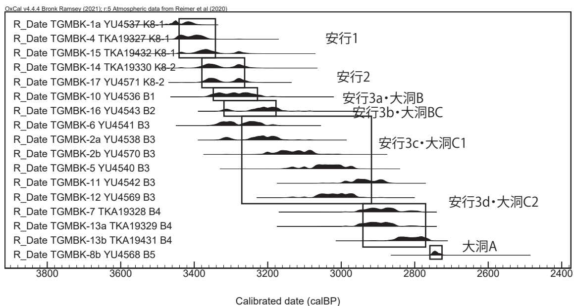
第6図 刈沼遺跡土器付着物の型式・時期別の較正年代
