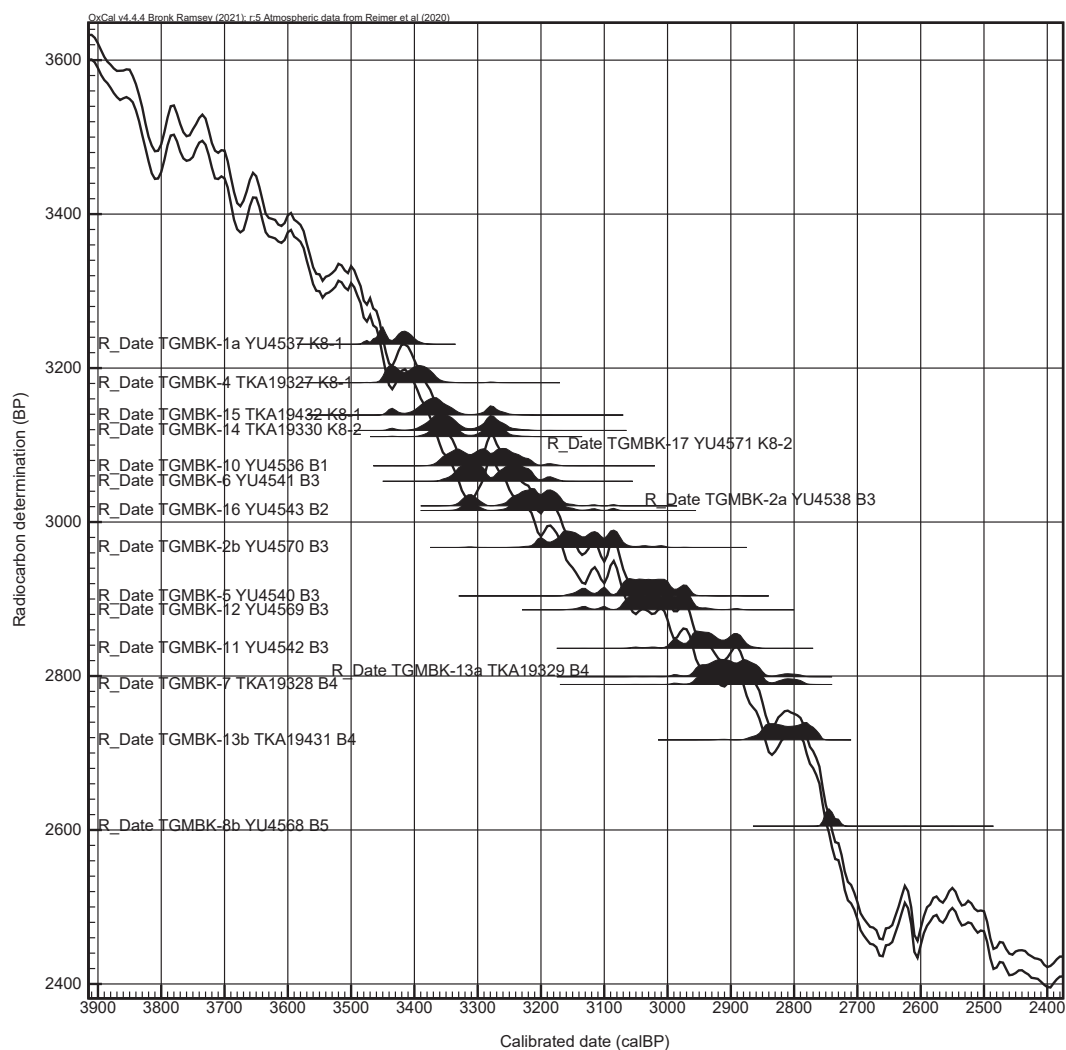
第7図 刈沼遺跡土器付着物の測定値と較正曲線 IntCal20
