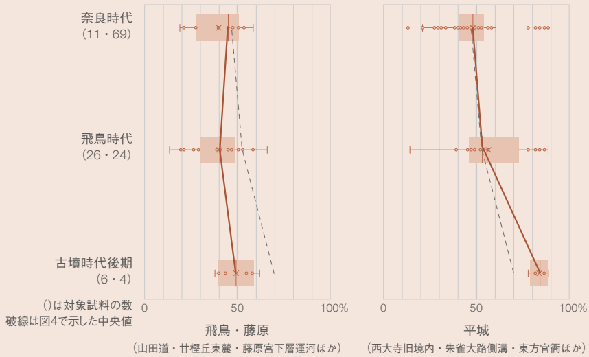
図5 木本花粉の割合変化の比較
