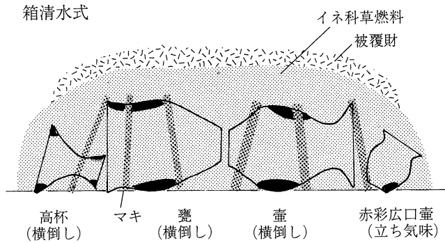
箱清水式
