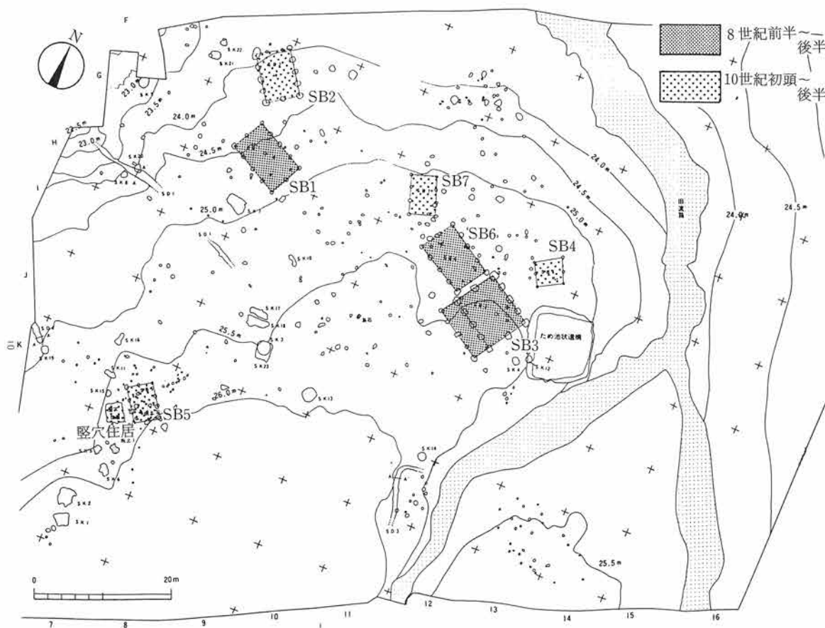
第22図 岩野下遺跡遺構配置図(県教委1987aを一部改変)
