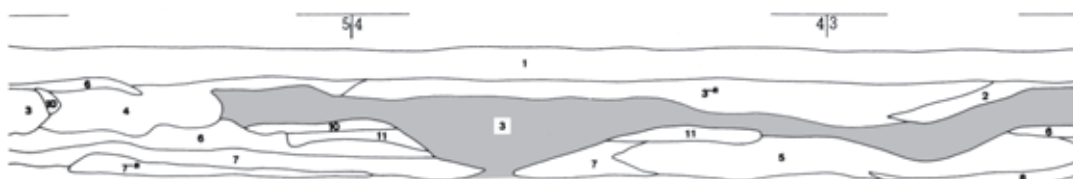
第13図 前田遺跡における噴砂脈 [川上2002] S=1:60 中央の3層が噴砂。
