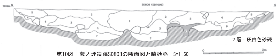
第10図 蔵ノ坪遺跡SD808の断面図と噴砂脈 S=1:60
