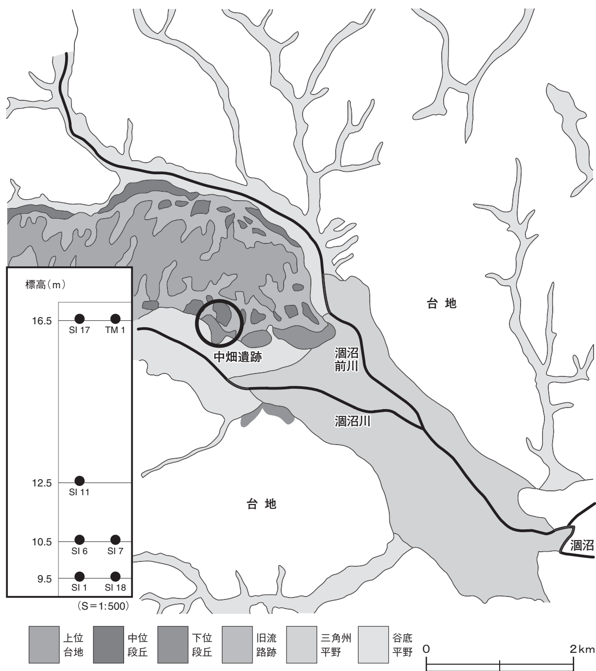
第247図 地形区分図（土地分類基本調査「石岡」1981年より）と古墳時代前期の遺構垂直分布図
