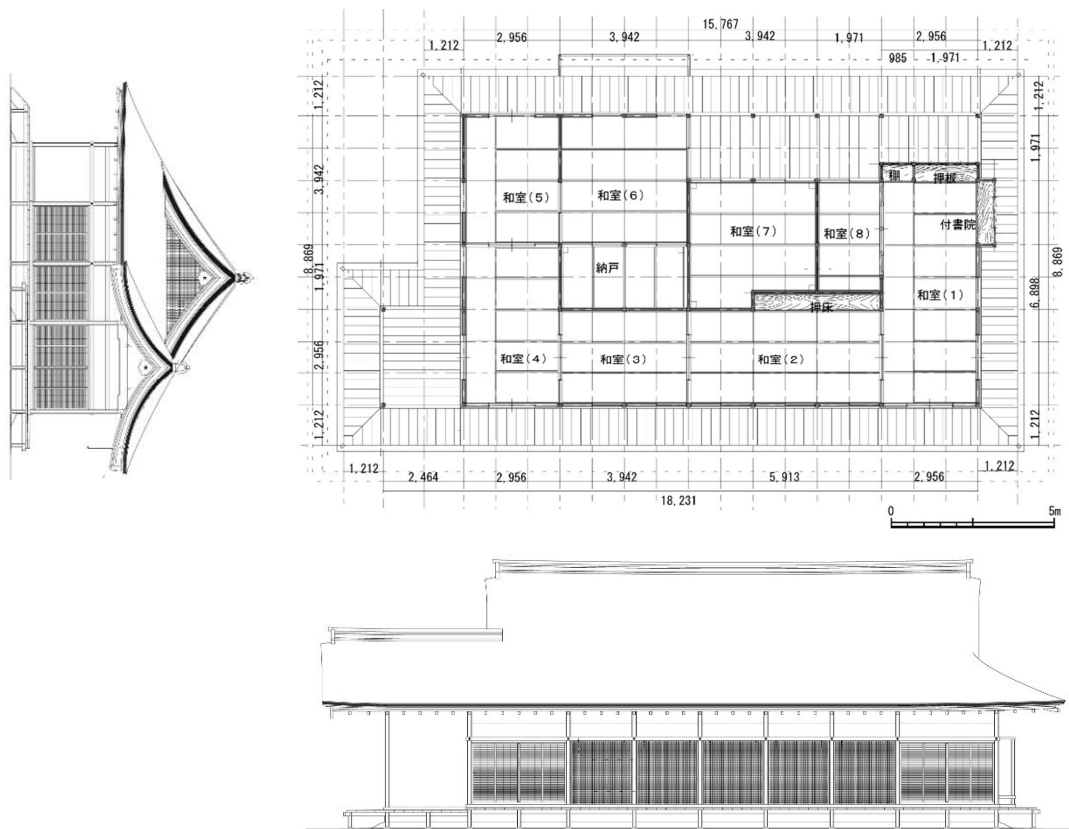
図 19 会所設計図
