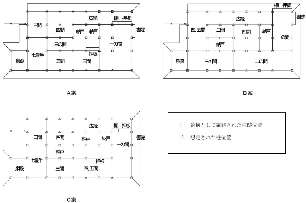
図 18 会所復元プラン
