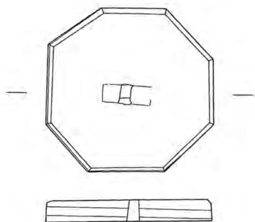
图2 台座実測図 (1:4)
