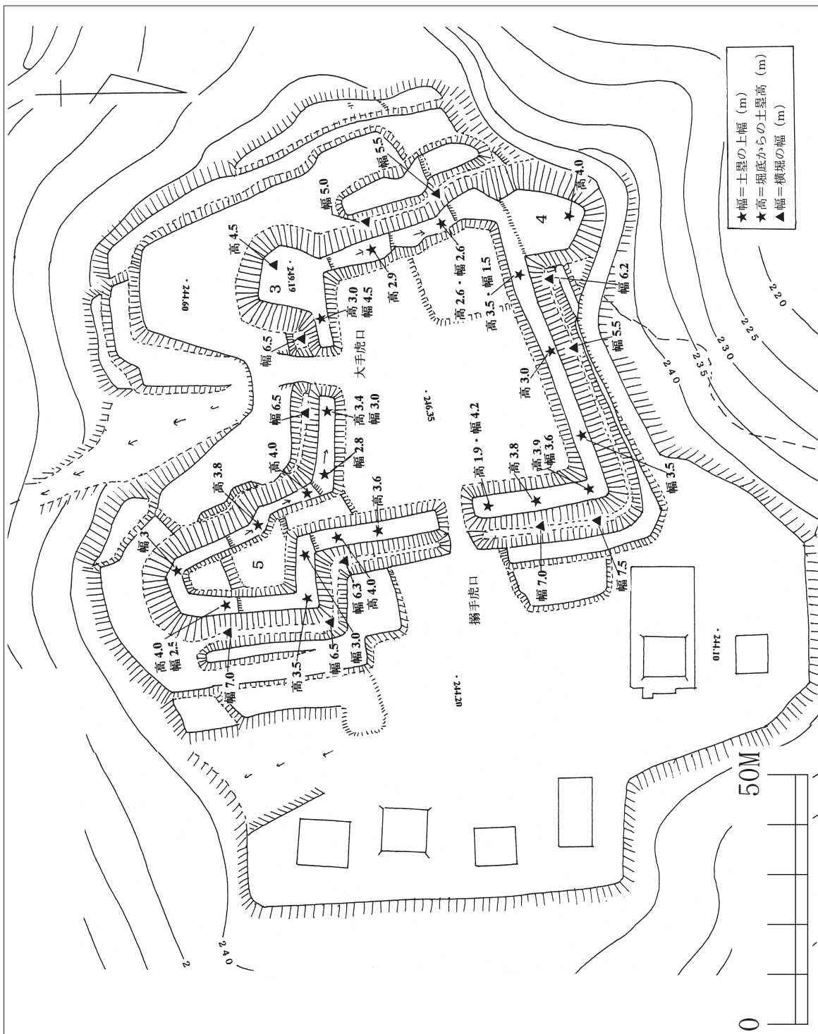
第2図 秀吉本陣の土塁と横堀の計測値
