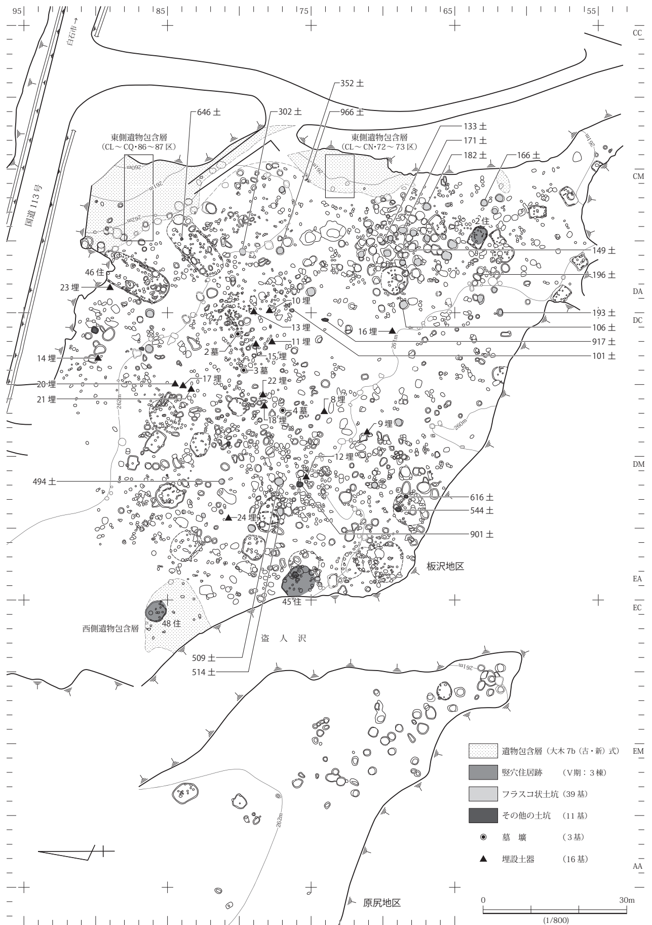
図10 小梁川遺跡Ⅳ～Ⅴ期（大木7b(古・新)式)の遺構配置
