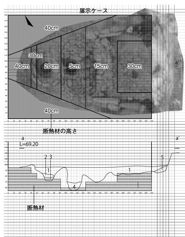
第7図 断熱材の切断仕様書
