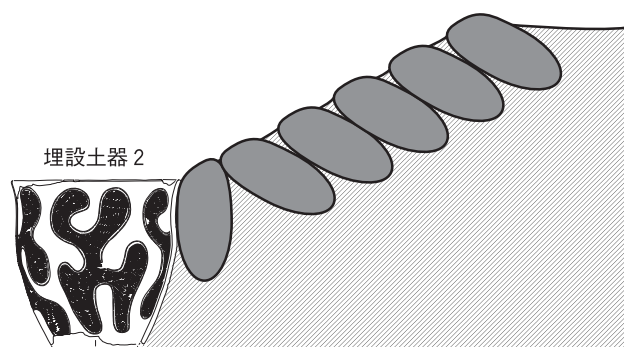
第25図 複式炉石組部断面の模式図（前庭部側から）
