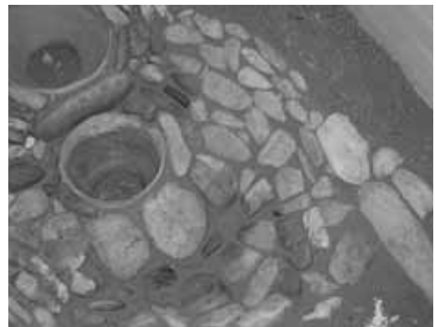
第23図 複式炉の石組部（復元）
