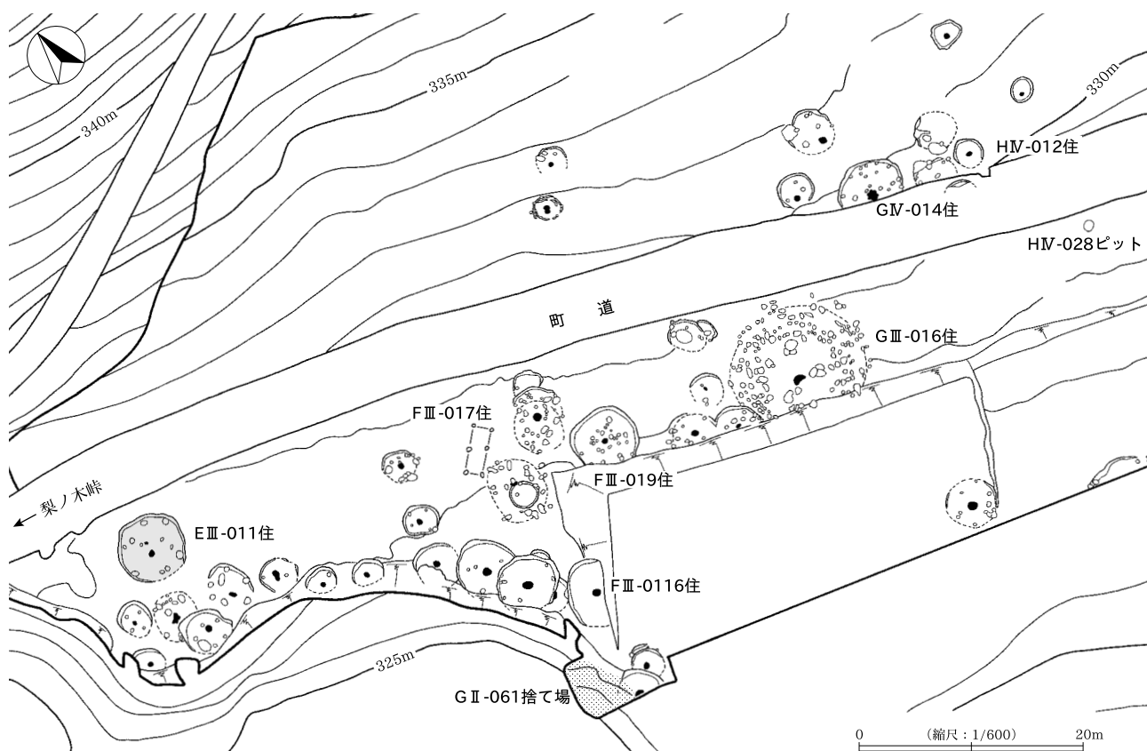
図2 曲田Ⅰ遺跡西側調査区遺構配置図
