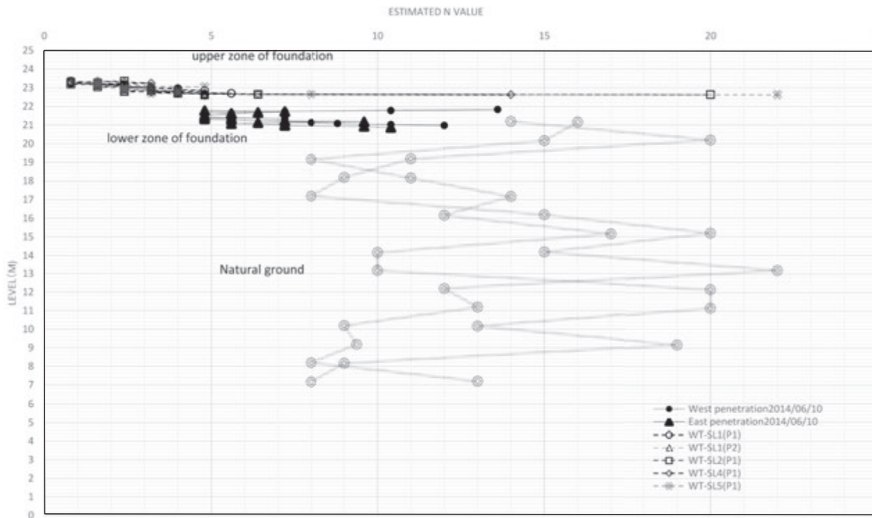
Fig. 7: N values
