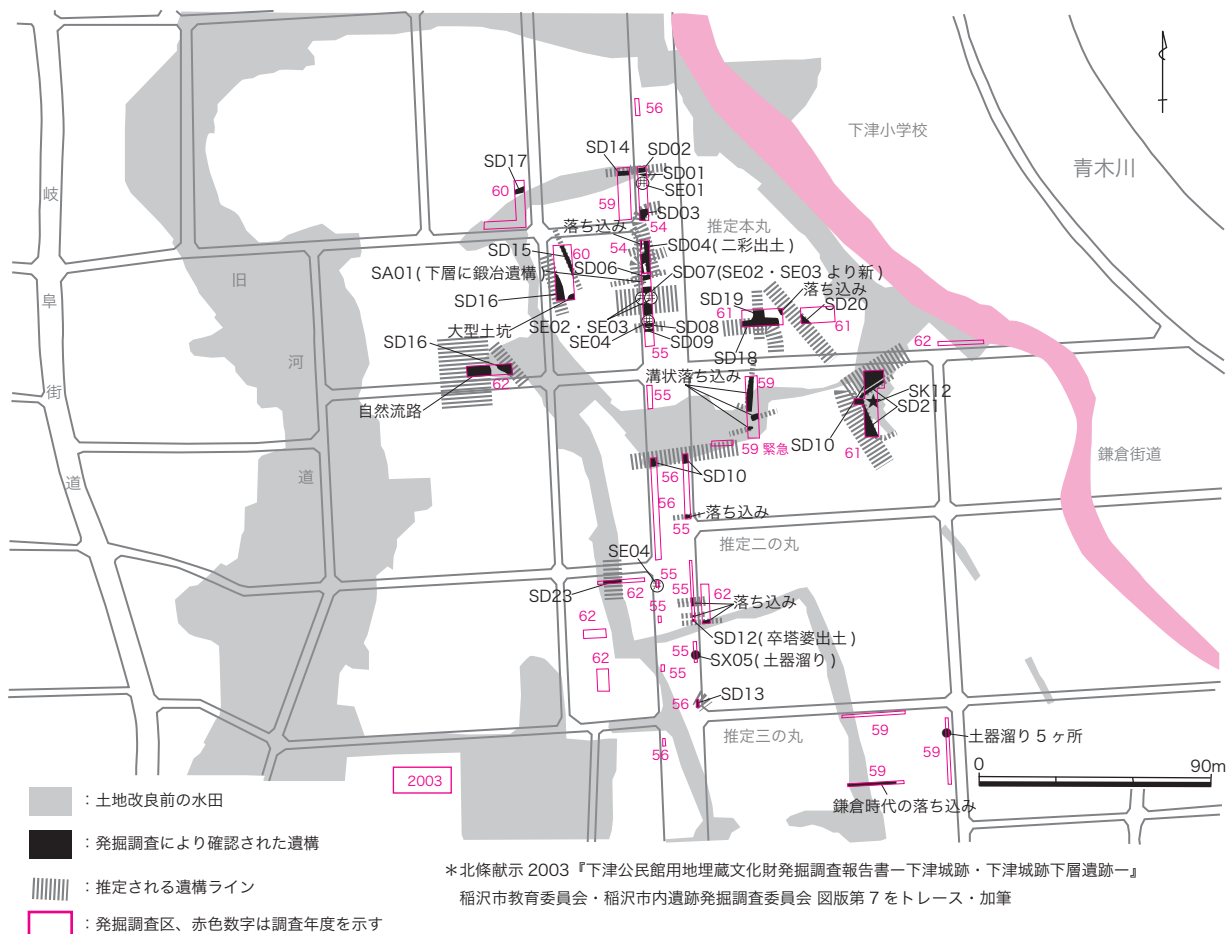
図8 下津城跡主要遺構配置図 (1:3,000)
