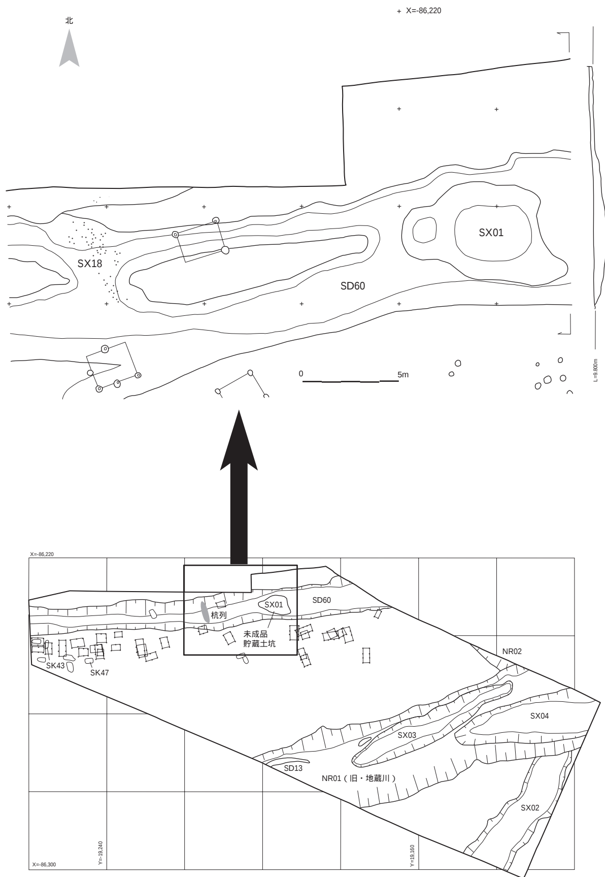
図3 勝川遺跡木製品製作関連施設遺構図 (S=1:1,000)(下) 同・拡大図 (S=1:200)(上)
