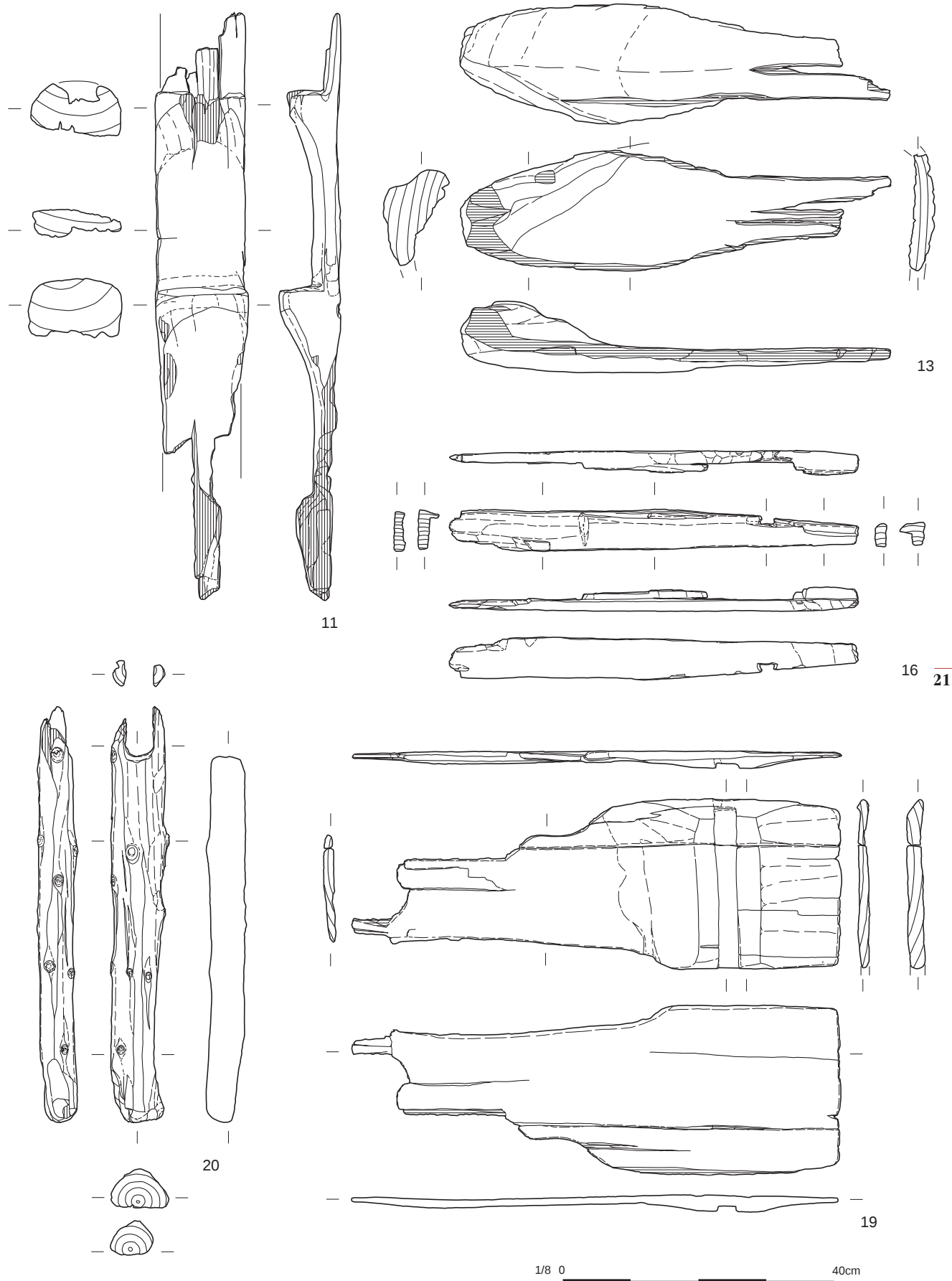
図 11 勝川遺跡出土木製品実測図(4) S=1 : 8
