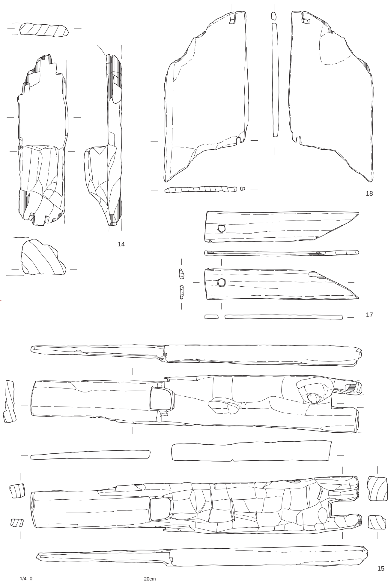
図12 勝川遺跡出土木製品実測図(5) S=1:4
