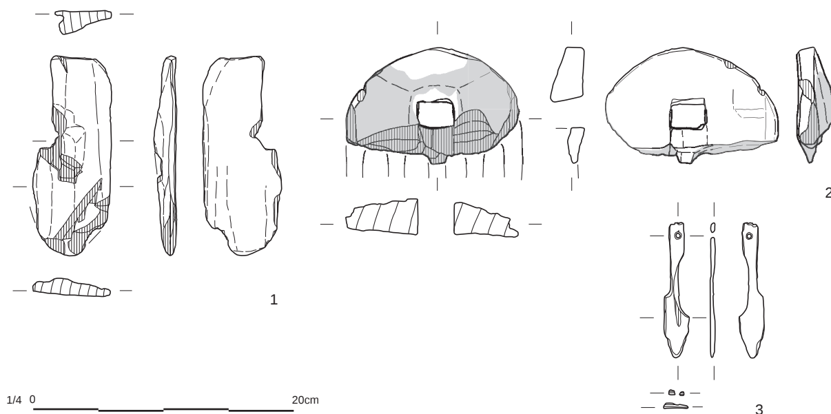
図8 勝川遺跡出土木製品実測図(1) S=1:4
