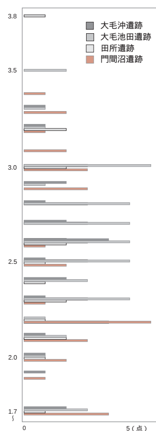
図6 門間沼遺跡ほか出土椀型滓の密度分布図
