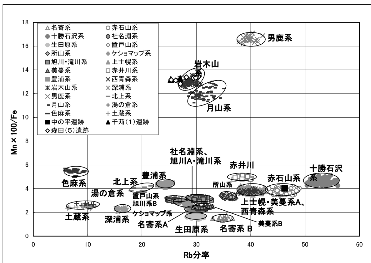
図 2 中の平遺跡、千苺 (1) 遺跡、森田 (5) 遺跡の判別図 (Rb 分率)
