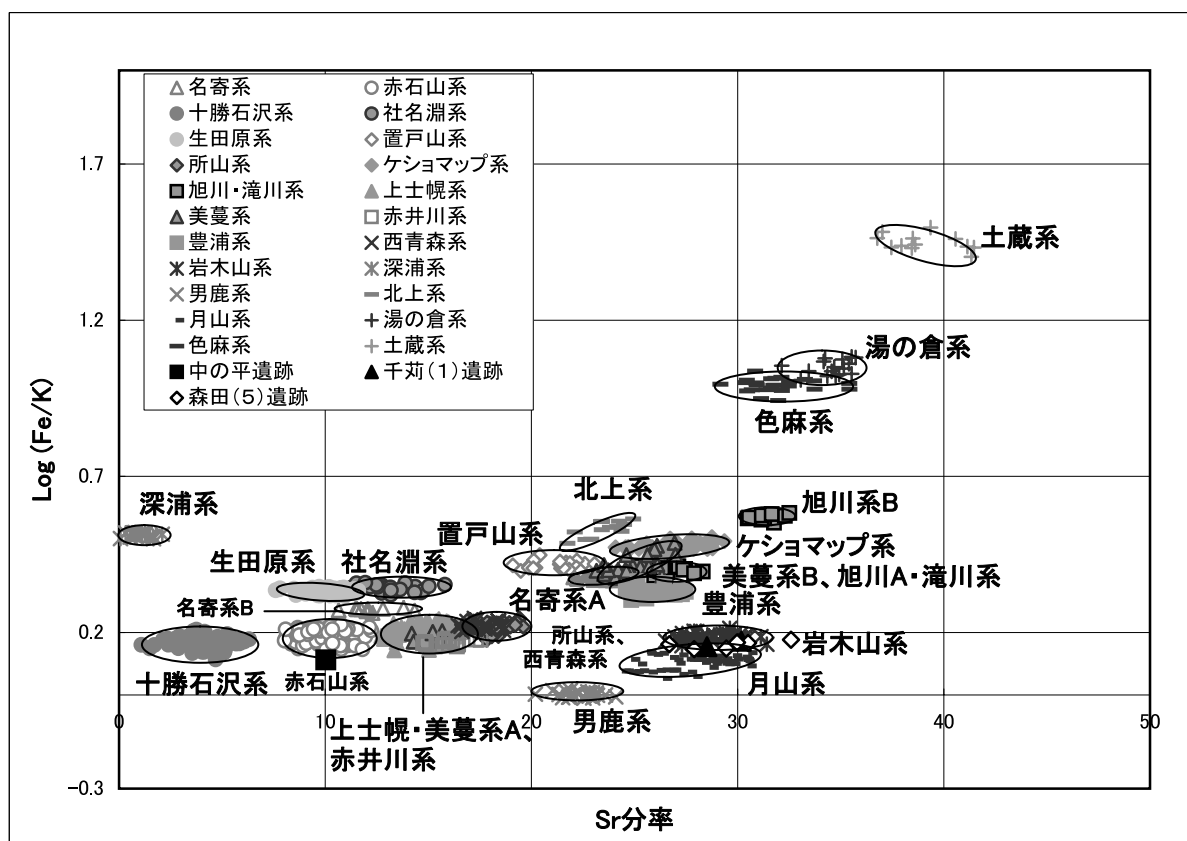
図 3 中の平遺跡、千苺 (1) 遺跡、森田 (5) 遺跡の判別図 (Sr 分率)
