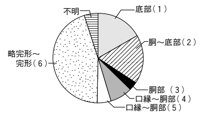
図3-3 残存比率
