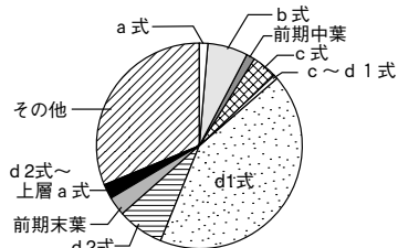
図3-2 形式別割合
