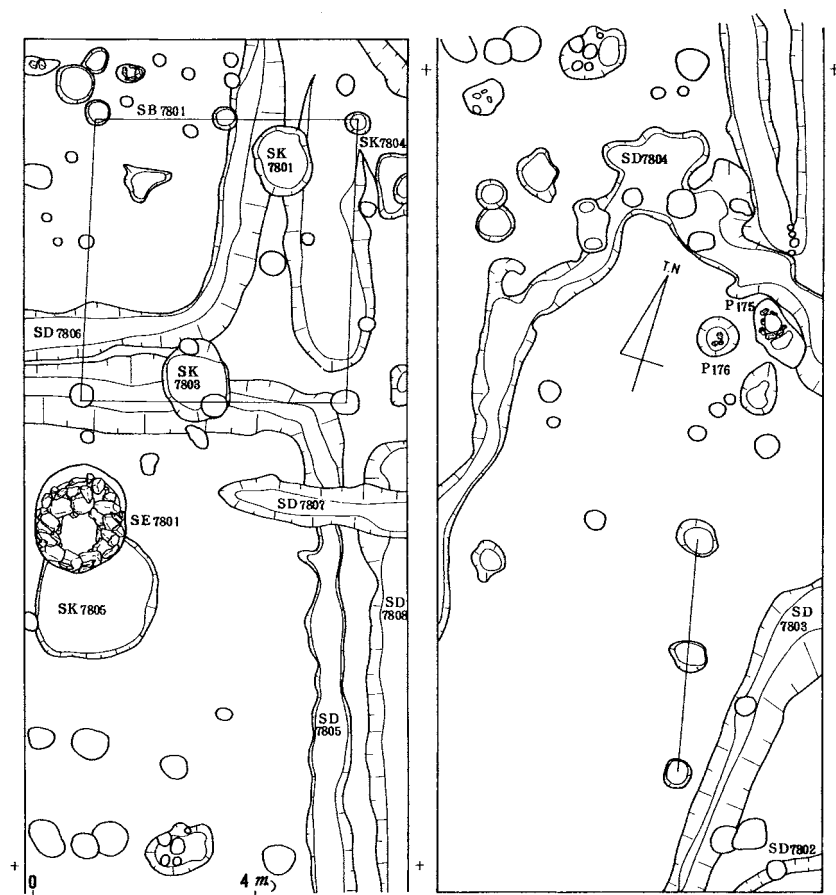
第10図 昭和53年度調査遺構実測図
