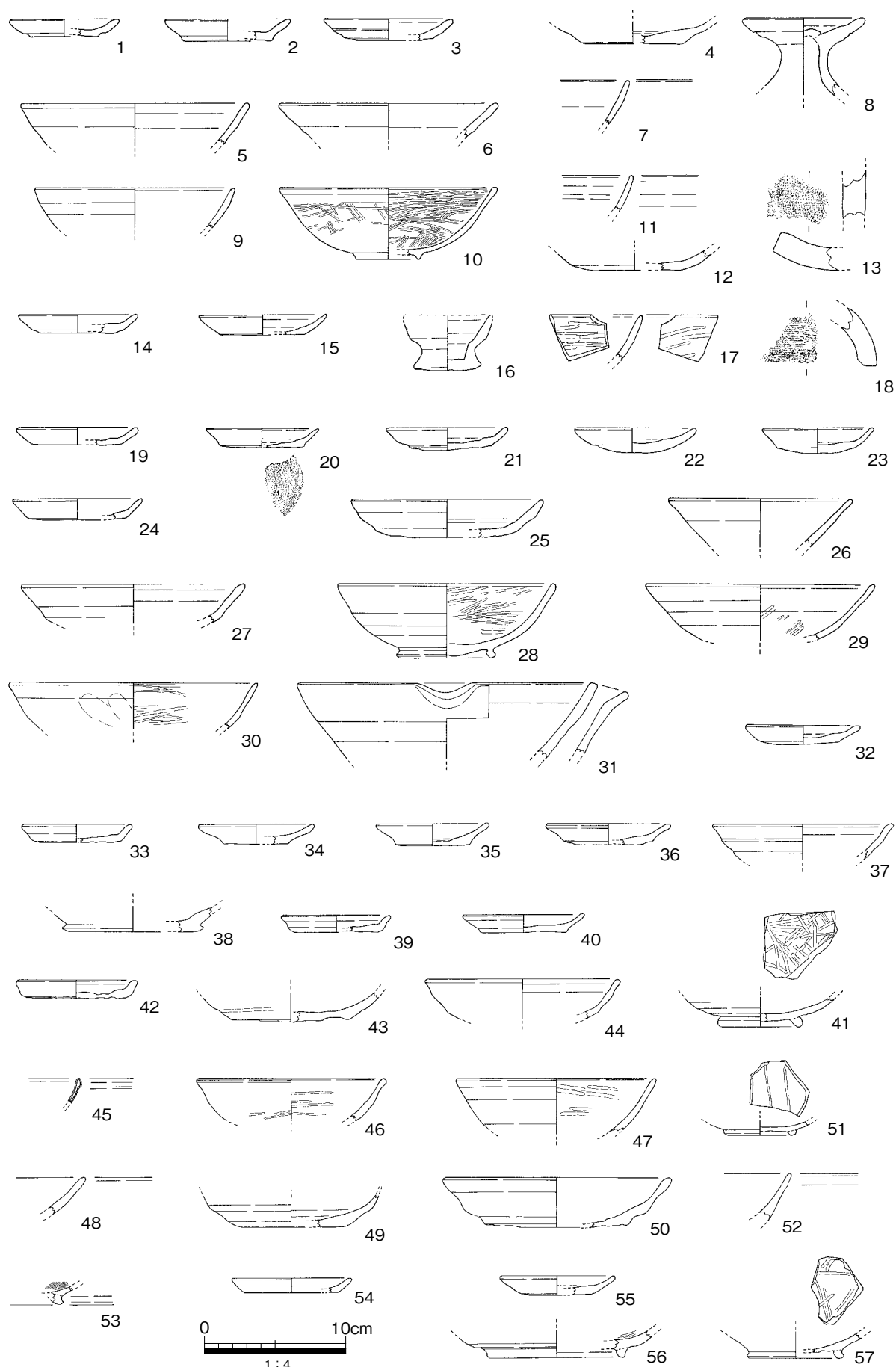
第12図 昭和54年度調査遺物実測図 1
