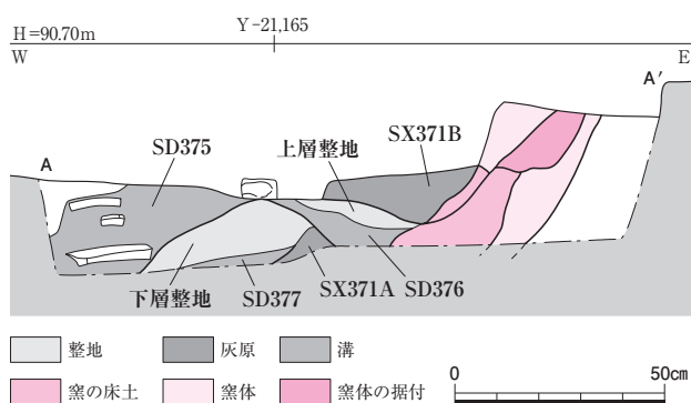
図263 SY370断面図 1 : 20
