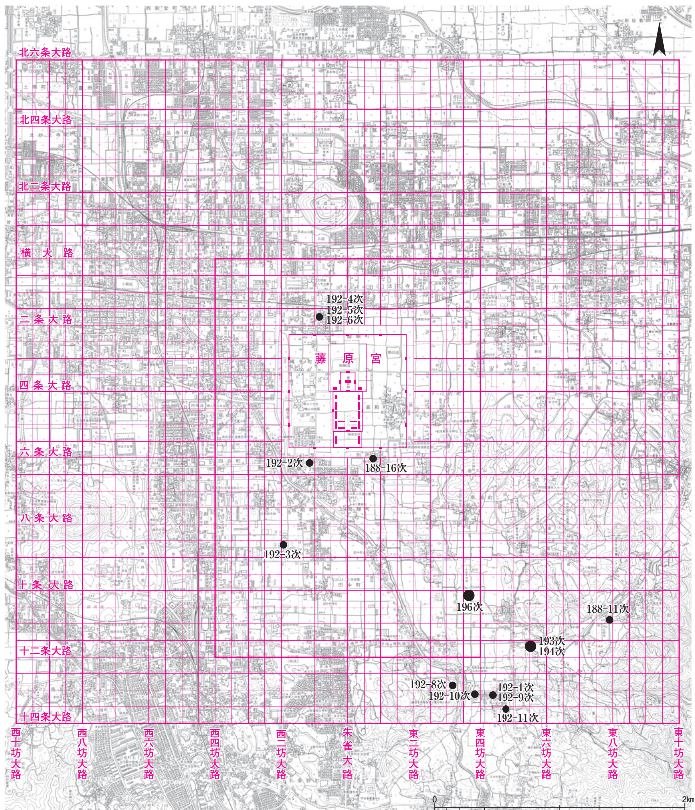
図108 藤原京発掘調査位置図 1 : 30000
