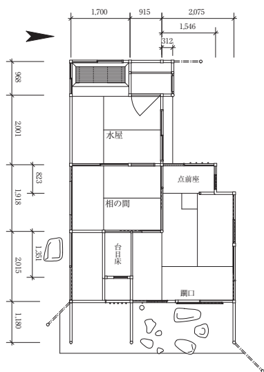
図44 八窓庵現況平面図 1 : 150
