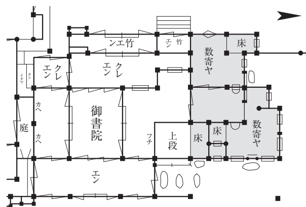
図47 隆遍代大乘院御殿建物指図の東北隅部分の描き起こし
