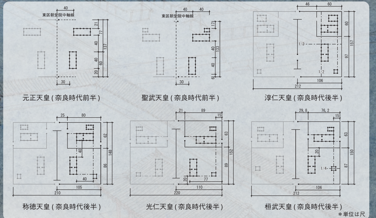
平城宮の大嘗宮遺構の規模と建物配置の変遷
