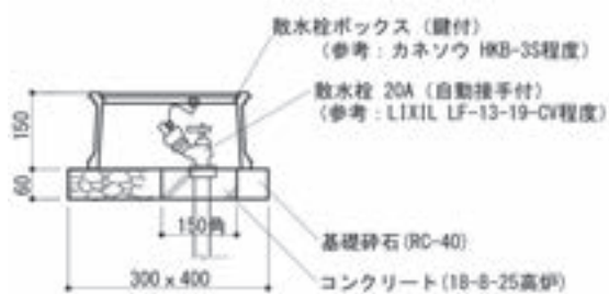
Fig.172 散水栓詳細図
