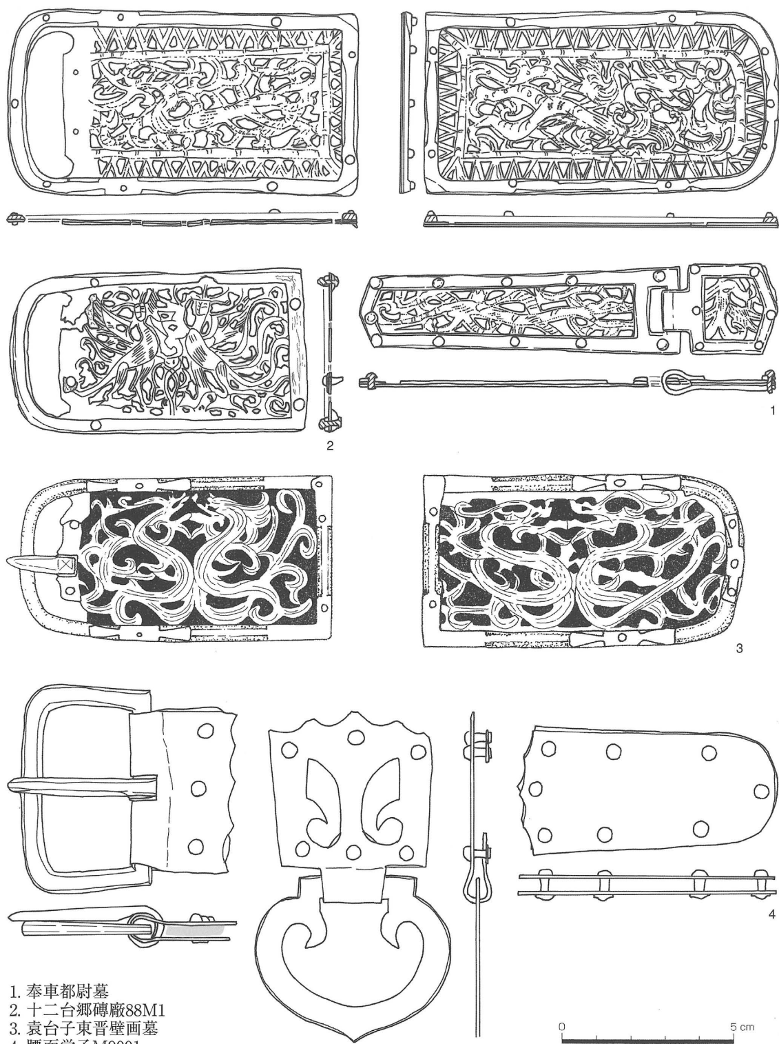
图1 三燕带金具（1）
