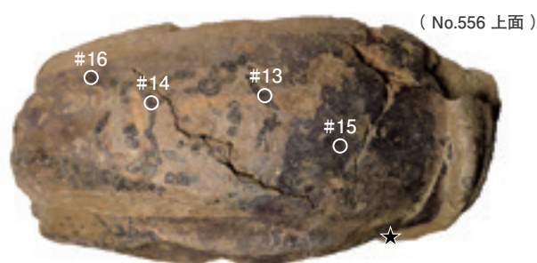
図100 ハンドヘルド型蛍光X線分析装置による調査での塑像No.556の測定位置(★は同一の部位を示す)
